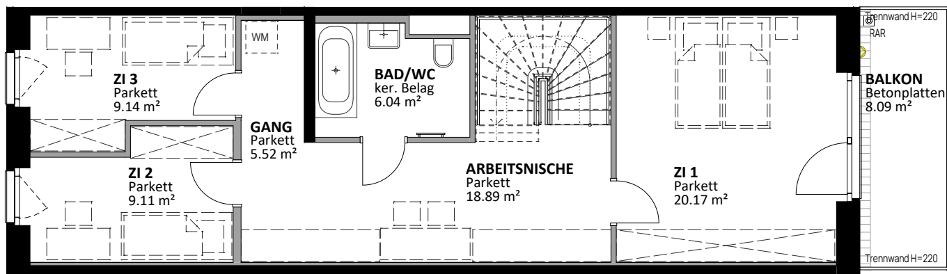
OG 1
